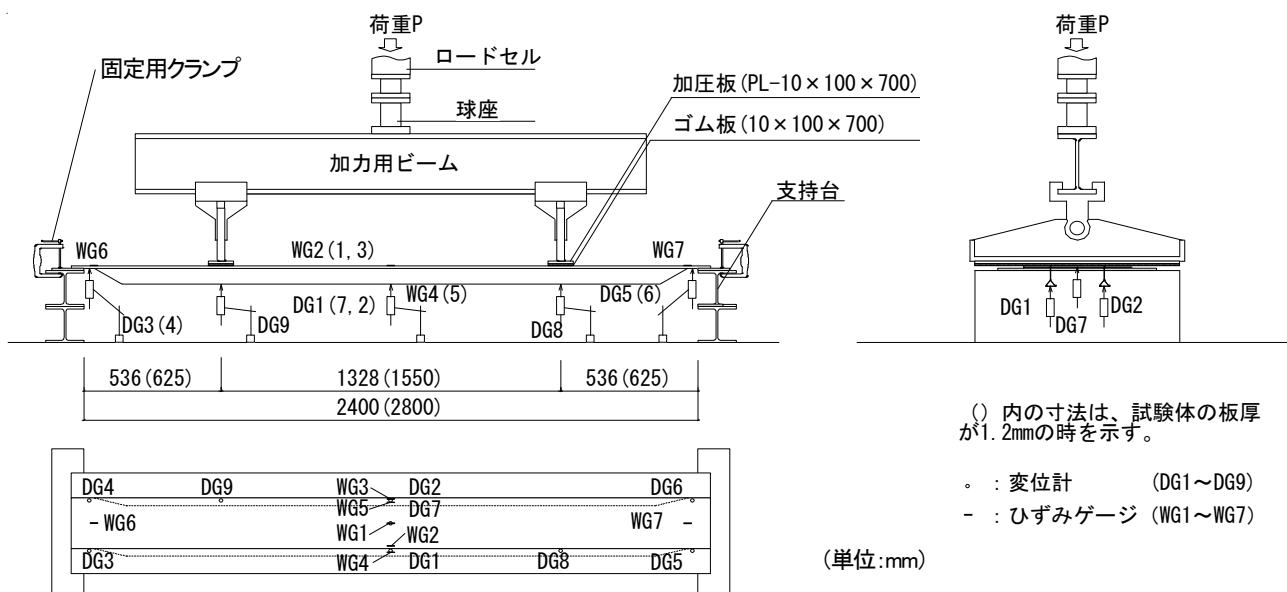
図－1 曲げ試験 試験方法
