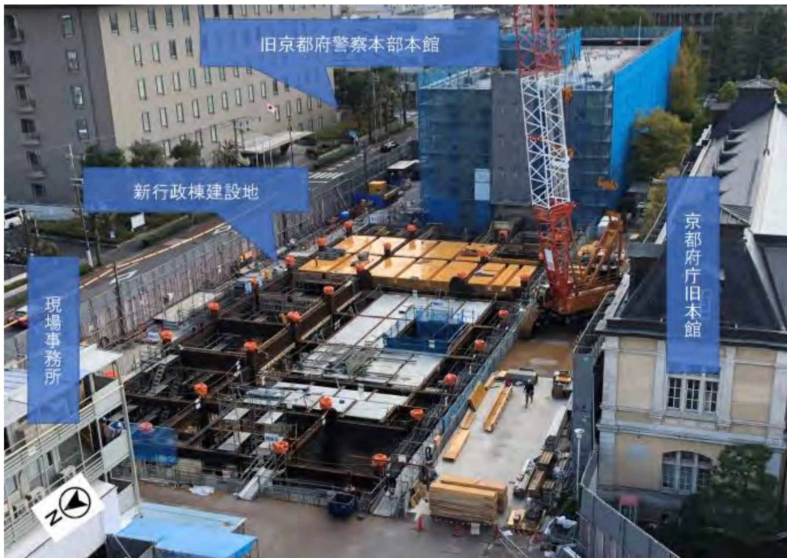
地下1階から1階床の配筋及び型枠工事（令和3年11月17日撮影）
