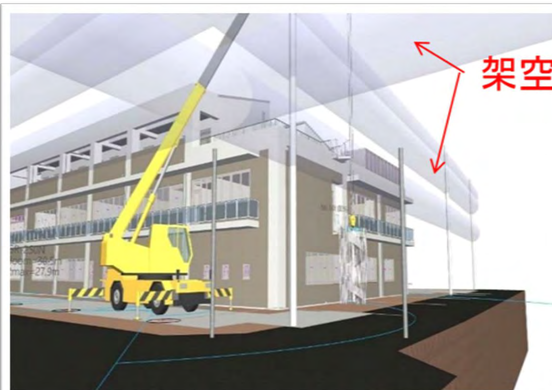
施工検討BIMモデル
