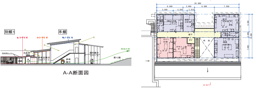
2階平面図
