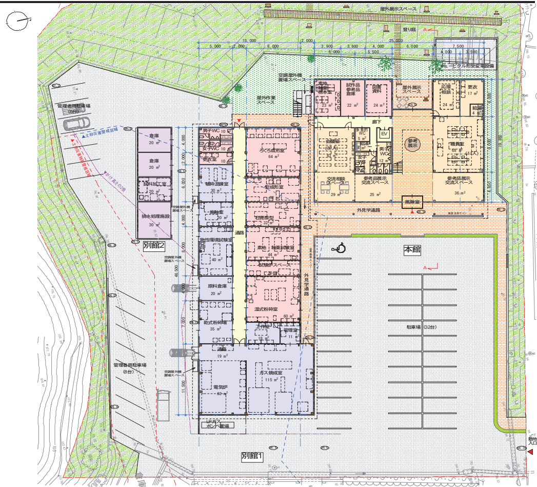
配置兼1階平面図
